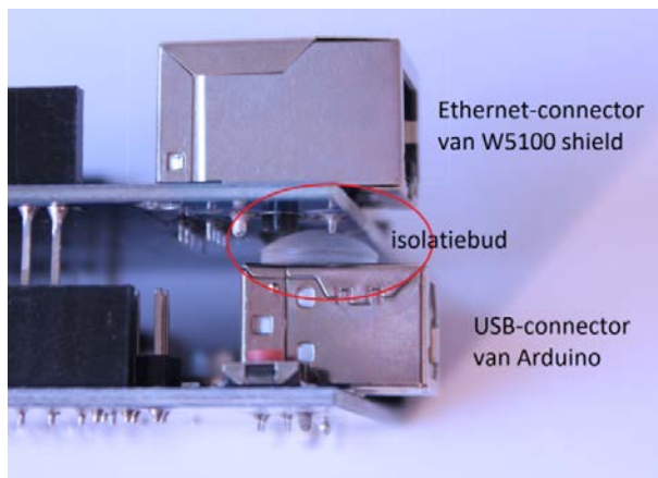
Afbeelding 14.6b – Isolatiebuis voorkomt contact tussen Ethernet-connector en USB-connector.
